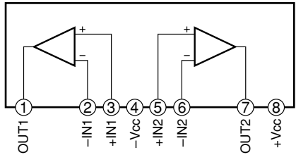
IC201: NJM2068L-D Dual OP-Amp
